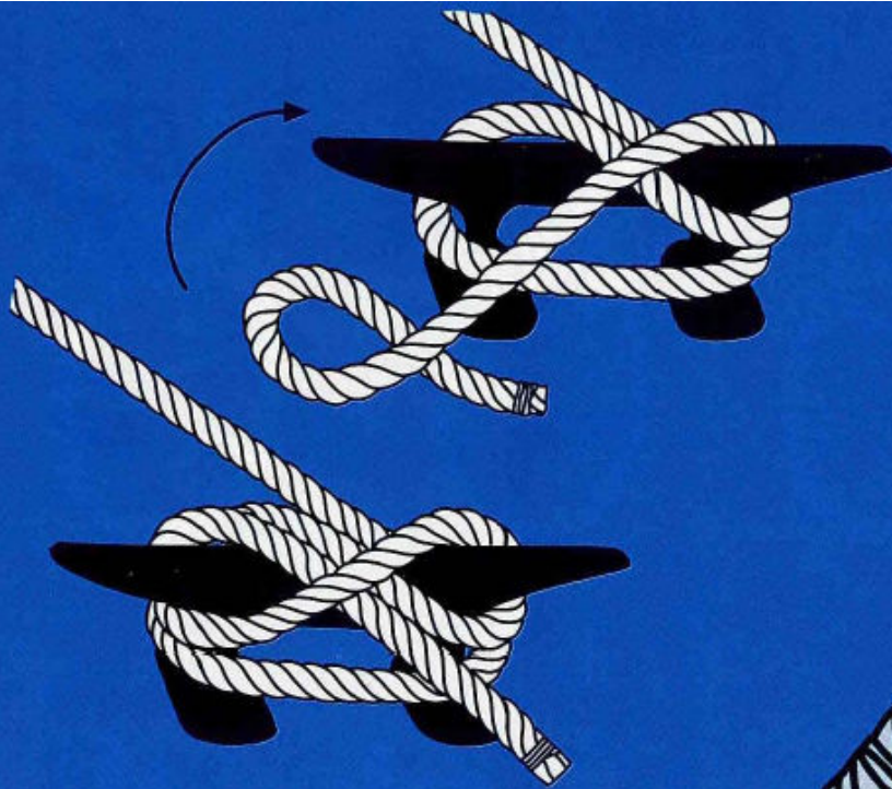
Belegen einer Klampe
